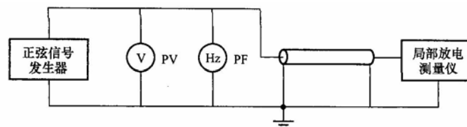
图1 局部放电测量仪频带测试接线图
