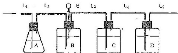
图 A.1 \text{ClO}_2 发生吸收装置图
