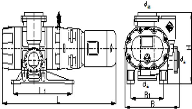
ZJ、ZJB、ZJL 型罗茨真空泵
