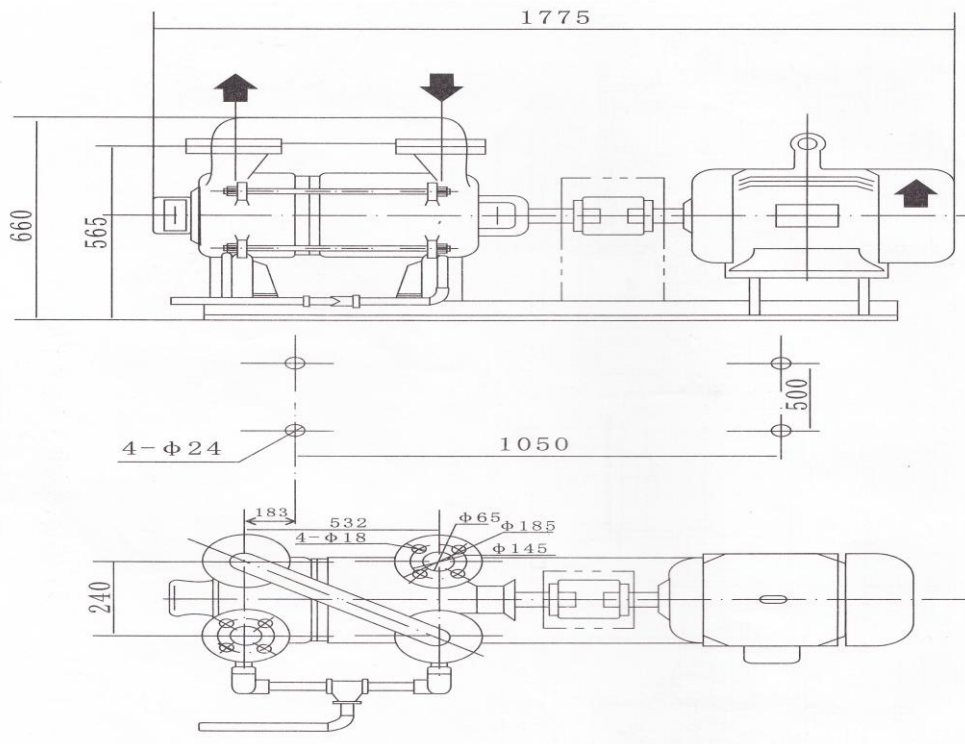
2SK-12 双级水环真空泵外形尺寸图
