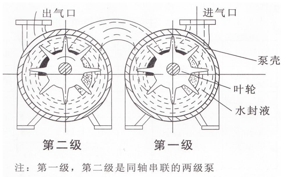
图 1 结构原理图
