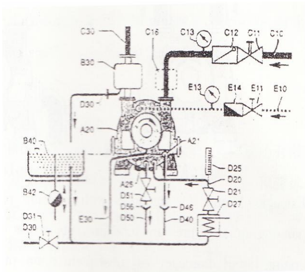
图 2c 工作液自动循环的连接示意图
