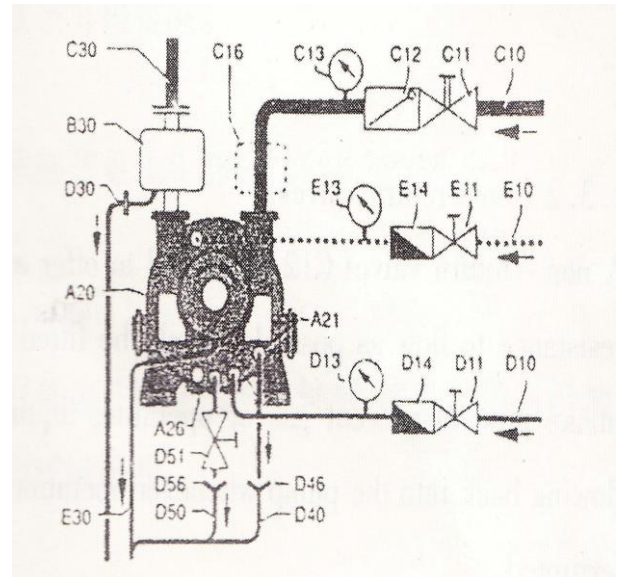
图 2b 带分离器的连接示意图
