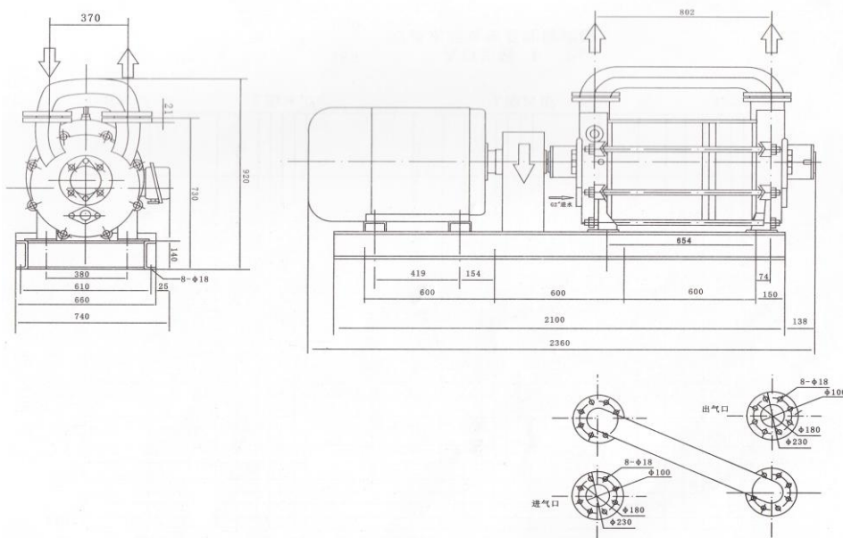
2SK-25 双级水环真空泵外形尺寸图
