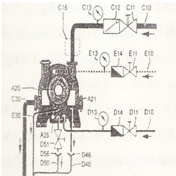
图 2a 不带分离器的连接示意图
