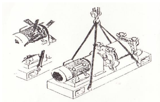
图 4 吊装示意图
