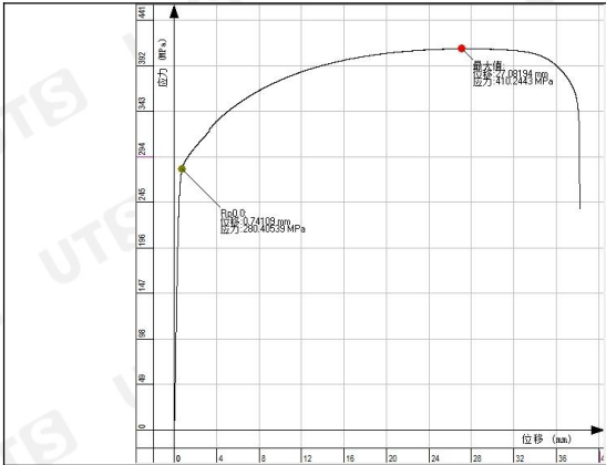
4-2-C 测试曲线(应力-位移)
