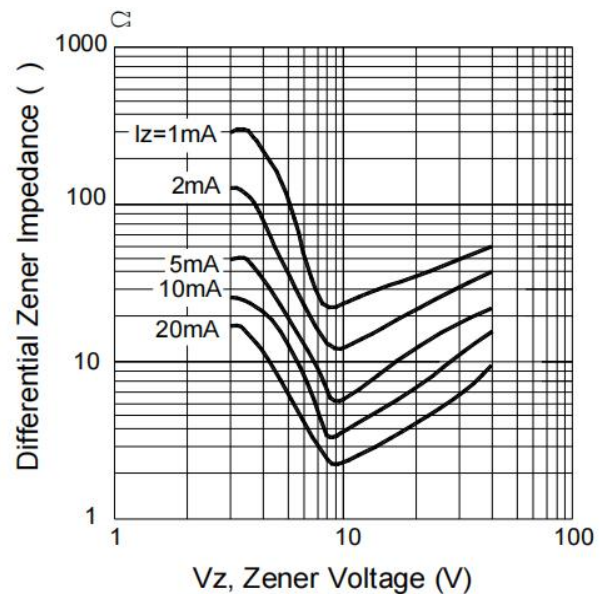
Fig. 4 Typical Zener Impedance vs. Zener Voltage
