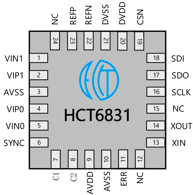
Figure 2-1 HCT6831 芯片引脚图
