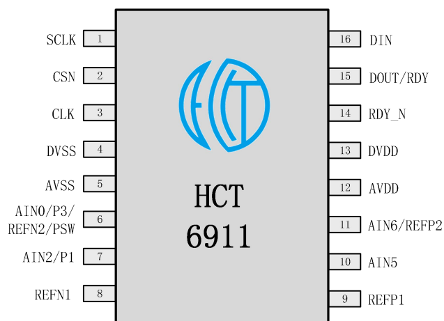
Figure 2-1 HCT6911 引脚分布图
