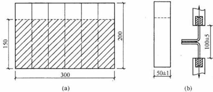
图 D. 2. 1 卷材—卷材剥离强度试样及试验
