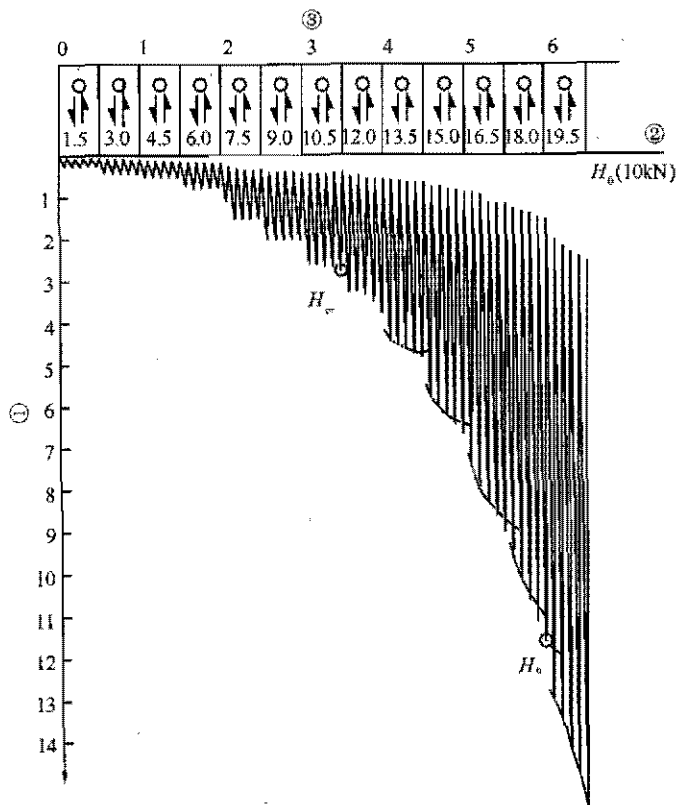
图 S.0.10-1 H_e-t-X_0 曲线
