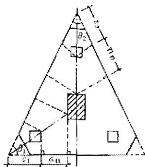
图 8.5.19-3 三角形承台角桩冲切验算
