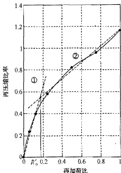
图 12 再压缩比率与再加载比关系
