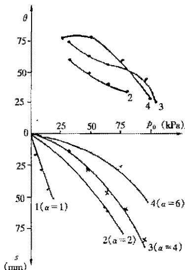
图 6 室内模型试验 p-s 曲线 p-\theta 曲线
