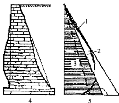
图 24 墙体变形与土压力
