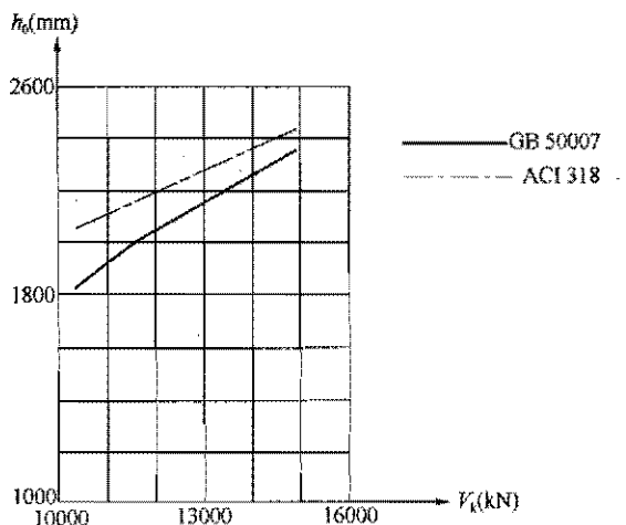
图 52 柱边剪切承台有效高度比较
