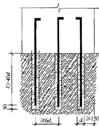
图 8.6.1 锚杆基础
