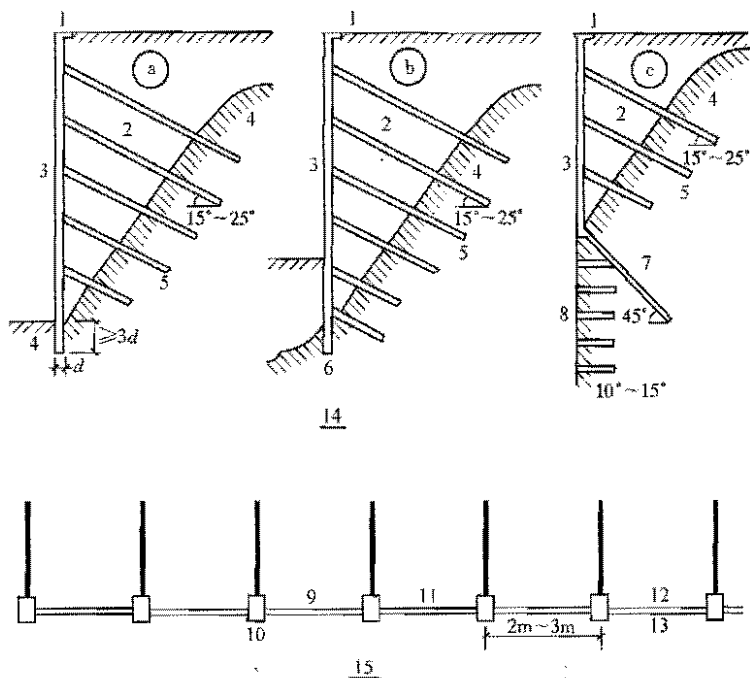
图 6.8.4 锚杆体系支挡结构
