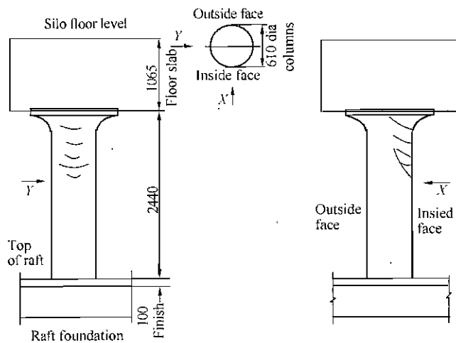
(b) 柱子裂缝示意
