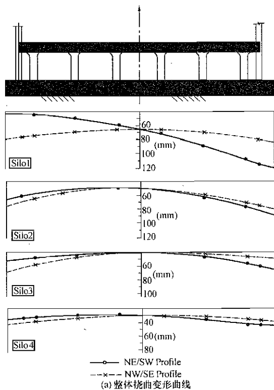
图 45 四幢地下仓库平板式筏基的整体挠曲变形曲线及柱子裂缝示意
