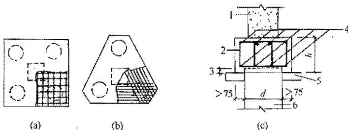
图 8.5.17 承台配筋
