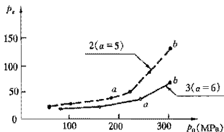
图 8 荷载板压力 p_0 与界面压力 p_z 关系
