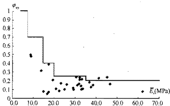
图 27 沉降计算经验系数与当量模量的关系
