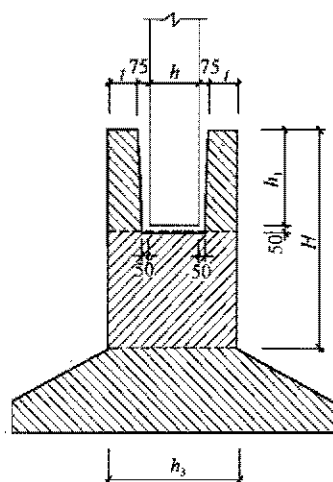
图 8.2.5-1 高杯口基础
