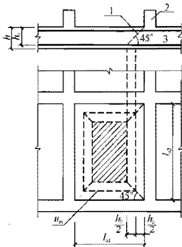
图 8.4.12-1 底板的冲切计算示意
