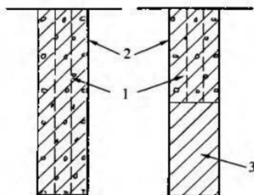
(a) 全复合散柔复合桩 (b) 分段复合散柔复合桩
