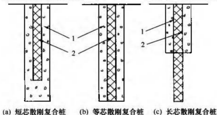
图 4.2.2 散刚复合桩构造示意图
