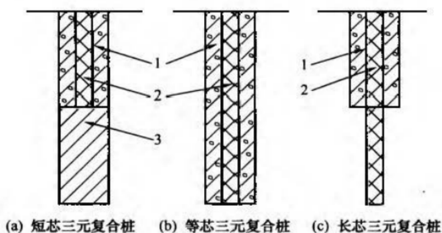
图 4.2.4 三元复合桩构造示意图
