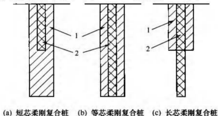
图 4.2.3 柔刚复合桩构造示意图
