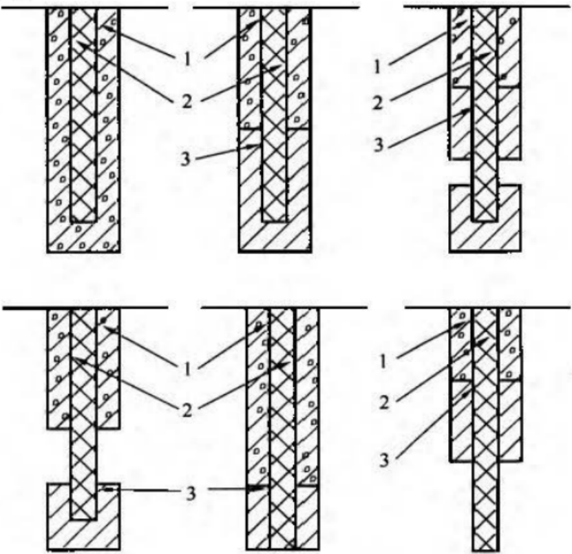
图3 三元复合桩其他构造形式示意图 1-散柔复合桩；2-刚性桩；3-柔性桩
