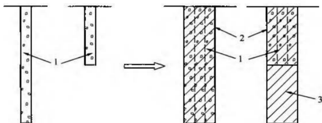
图 1 散柔复合桩施工过程
