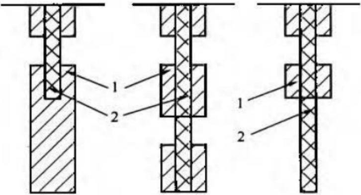
图2 柔刚复合桩分段复合构造示意图 1--柔性桩；2--刚性桩
