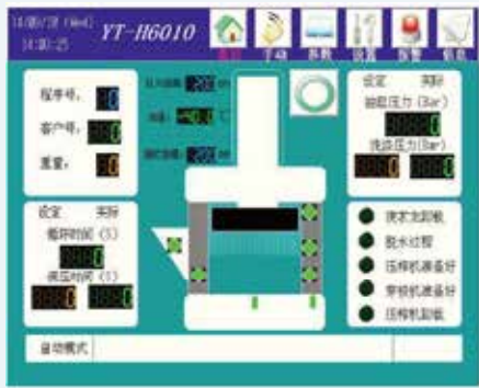
主控制界面主要用于设备运行状态的监控
