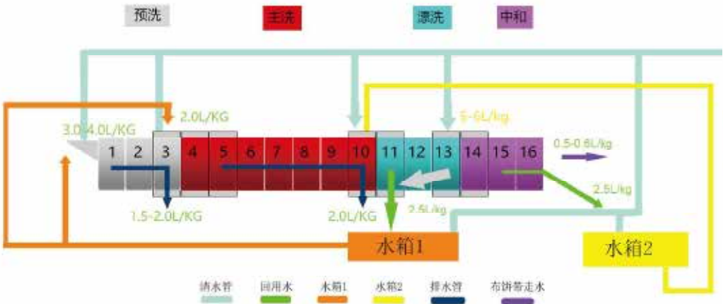
顺流漂洗介质流程图
