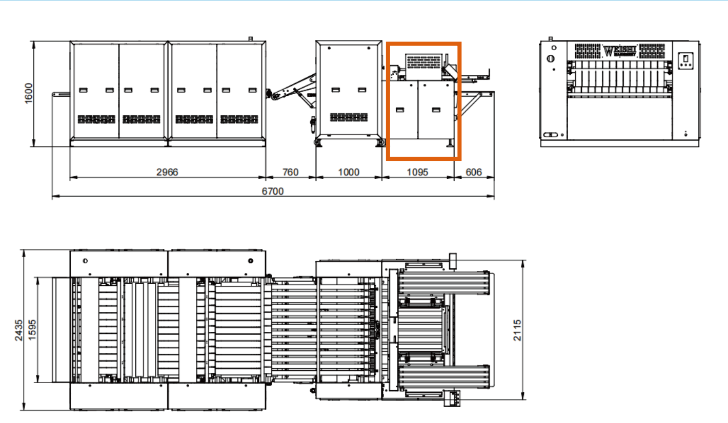
十字折尺寸图（可增加选项）
