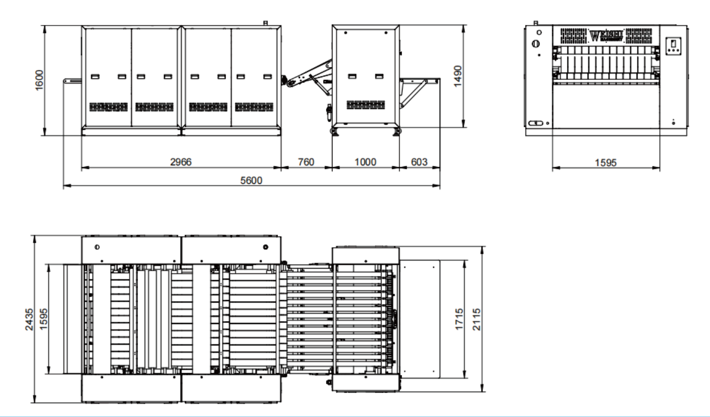
两横折尺寸图
