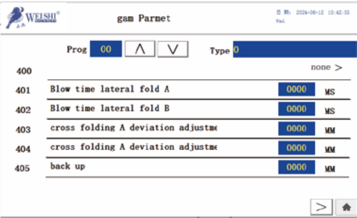
折叠机运行数据分析图（触摸屏）
