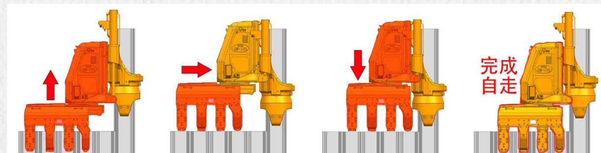
桩上自走步骤
