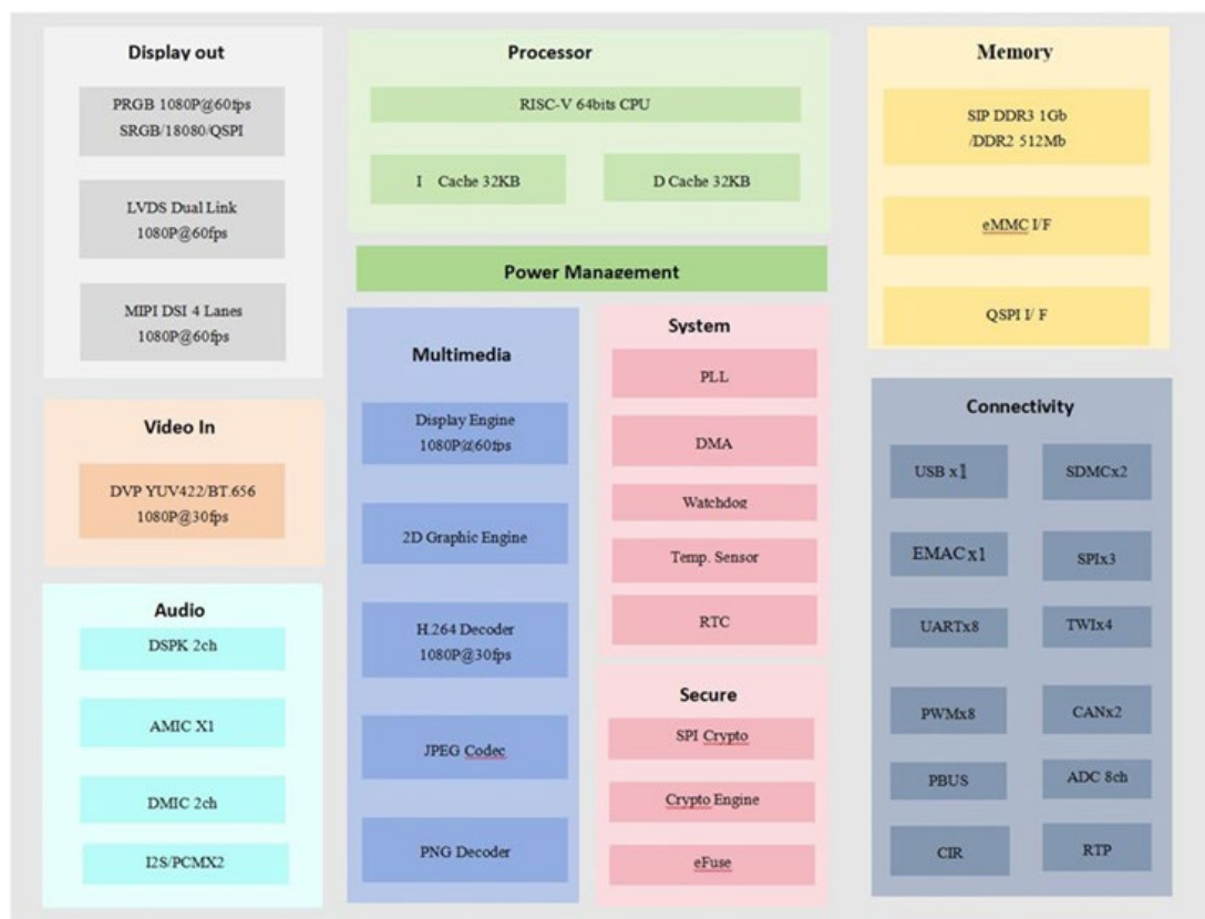
Fig.1 Internal Function Block Diagram (图 1 内部功能框图)
