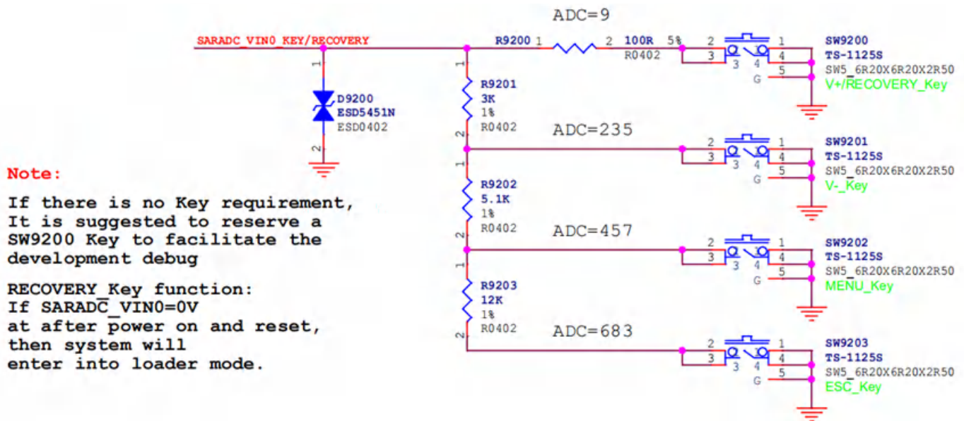
图15. ADC扩展按键参考设计图
