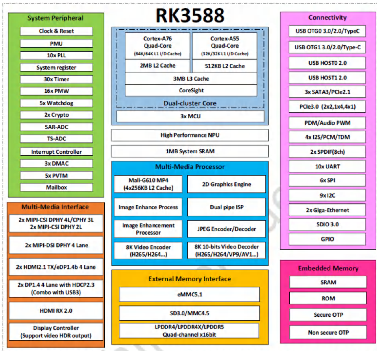
图1.RK3588模块框图
