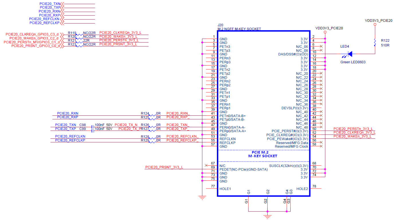
图10. PCIe2.0接口设计
