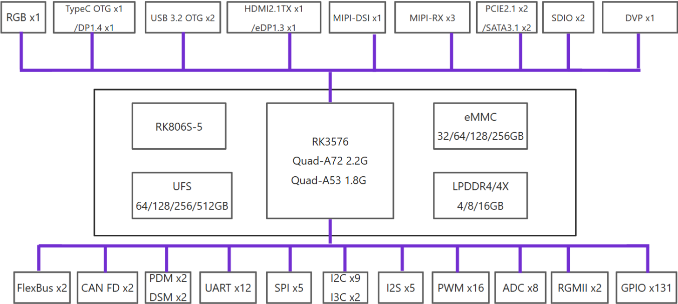
图2. IDO-SOM7608-V1功能框图
