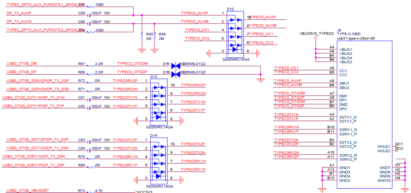
图20. TYPEC座子的ESD电路
