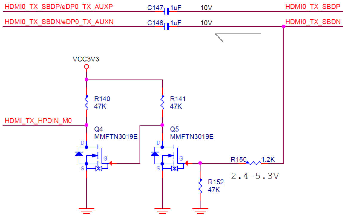
图24. SOM7608-V1 HDMI TX HPD电路
