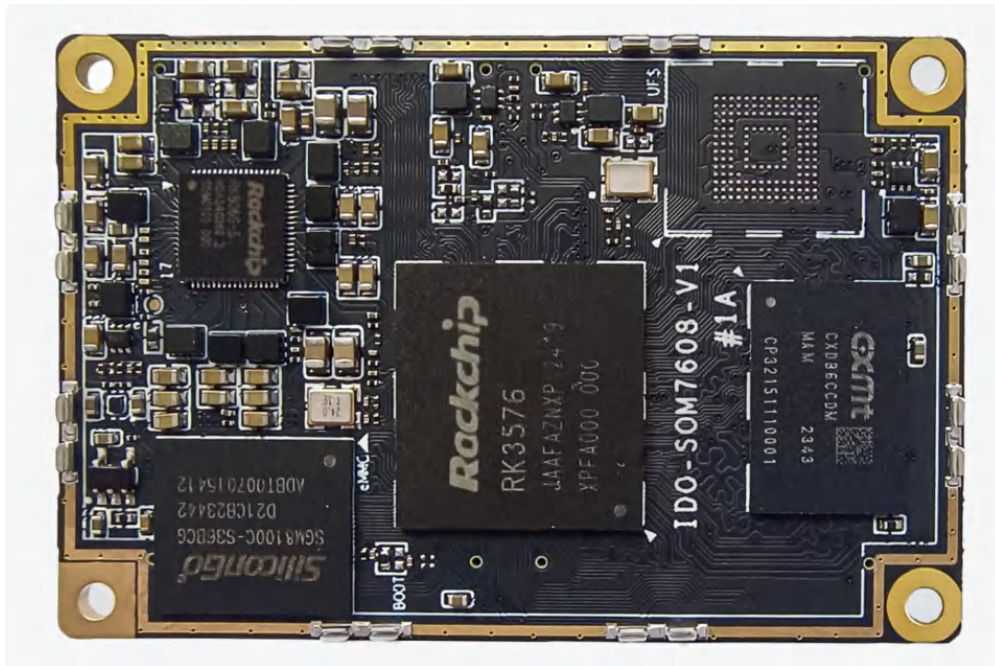
图3. IDO-SOM7608-V1核心板正面
