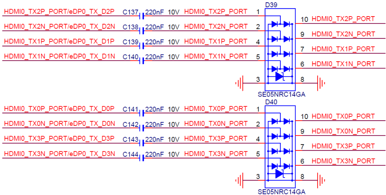
图21. SOM7608-V1 HDMI TX AC耦合电容外围电路
