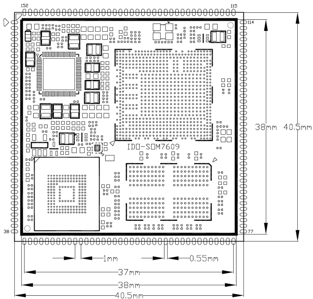
IDO-SOM7609-S1核心板背面尺寸，如下图所示：
