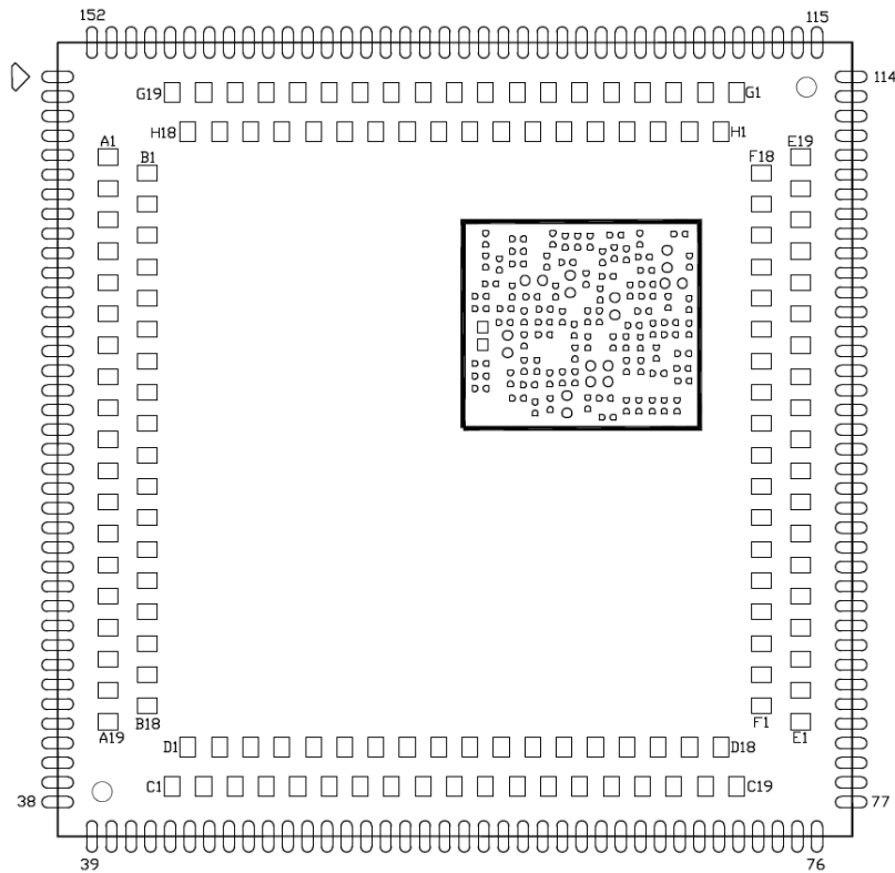
IDO-SOM7609-S1核心板PIN-OUT图，如下图所示：
