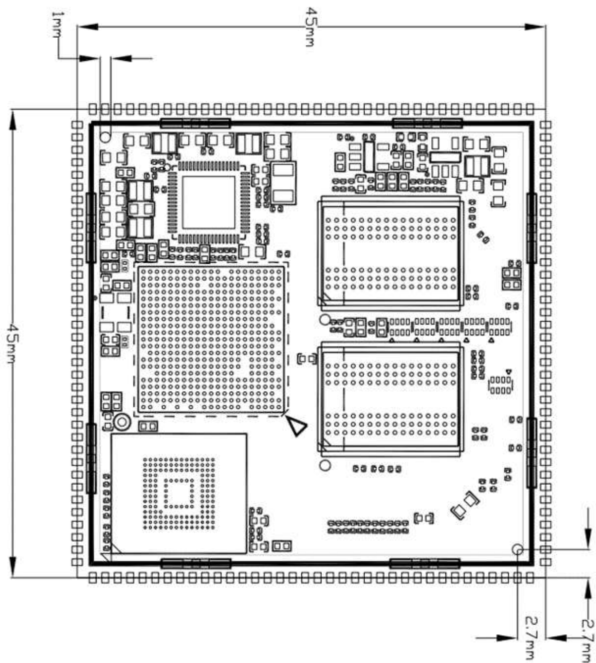
图5. IDO-SOM3020核心板正面尺寸
