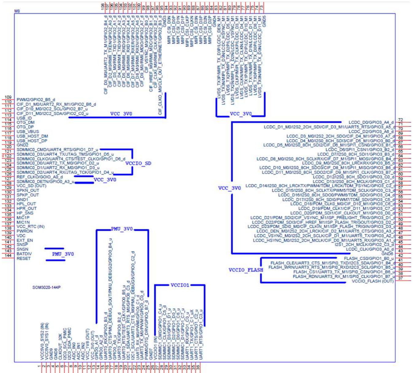
图7. IDO-SOM3020核心板引脚示意图
