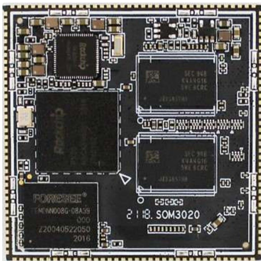
图3. IDO-SOM3020核心板正面
