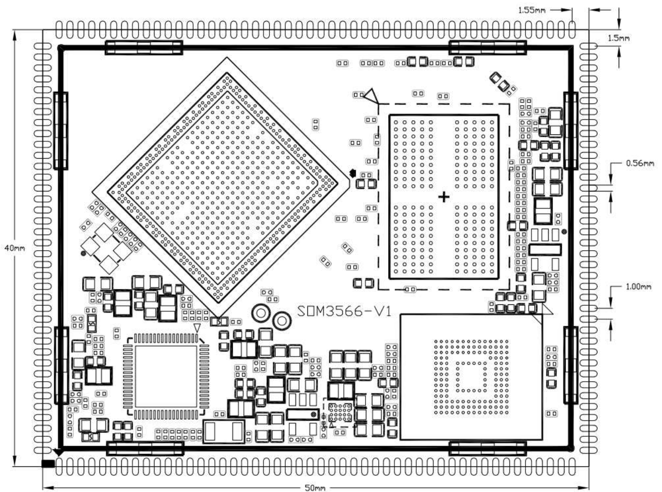
IDO-SOM3566-V1核心板背面尺面尺寸，如下图所示：
