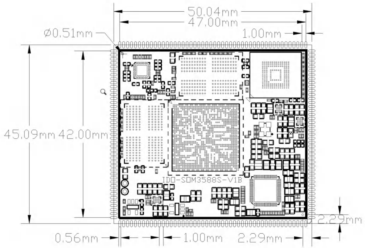
IDO-SOM3588S-V1核心板背面尺寸，如下图所示：
