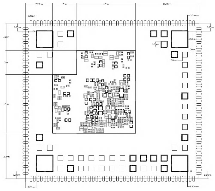
IDO-SOM3588S-V1核心板背面尺寸，如下图所示：
