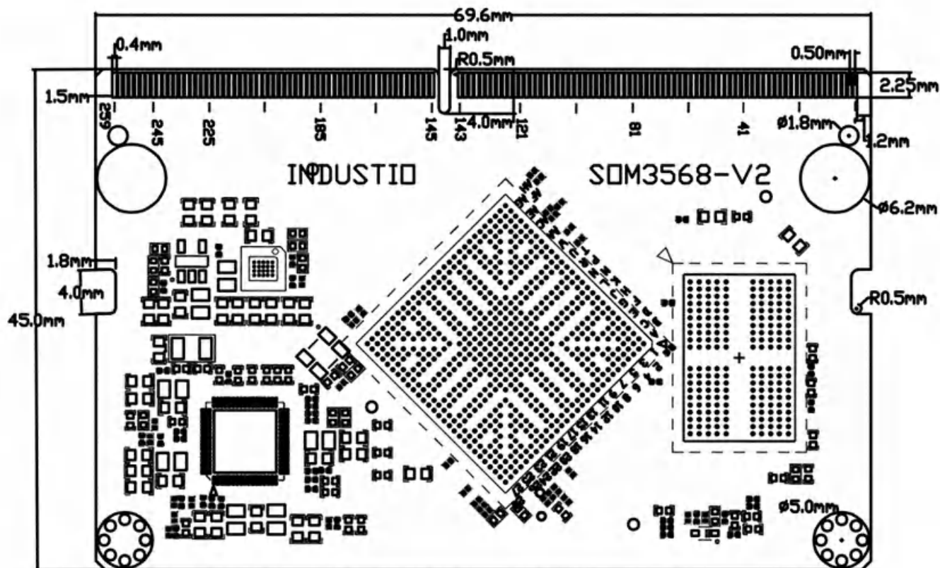
图5. IDO-SOM3568J-V2核心板正面尺寸
