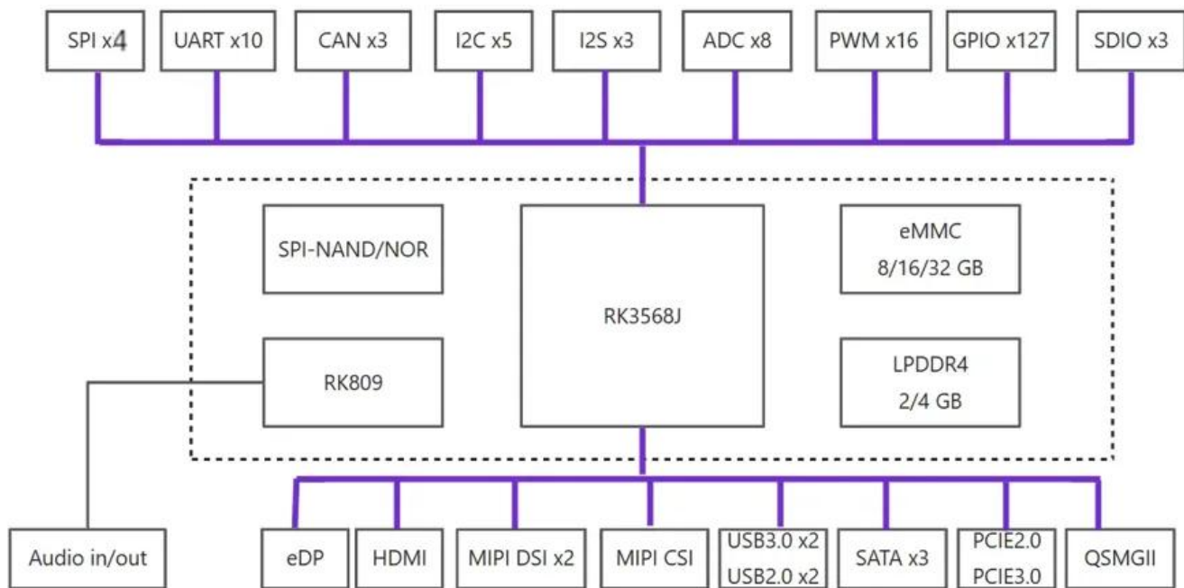
图2. IDO-SOM3568J-V2模块逻辑框图
