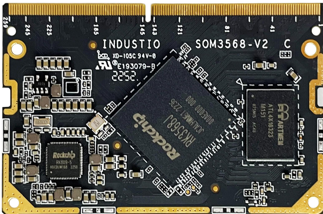
图3. IDO-SOM3568J-V2核心板正面
