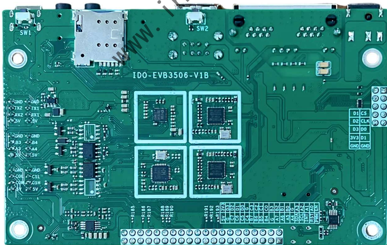
IDO-EVB3506-V1背面图，如下图所示：
