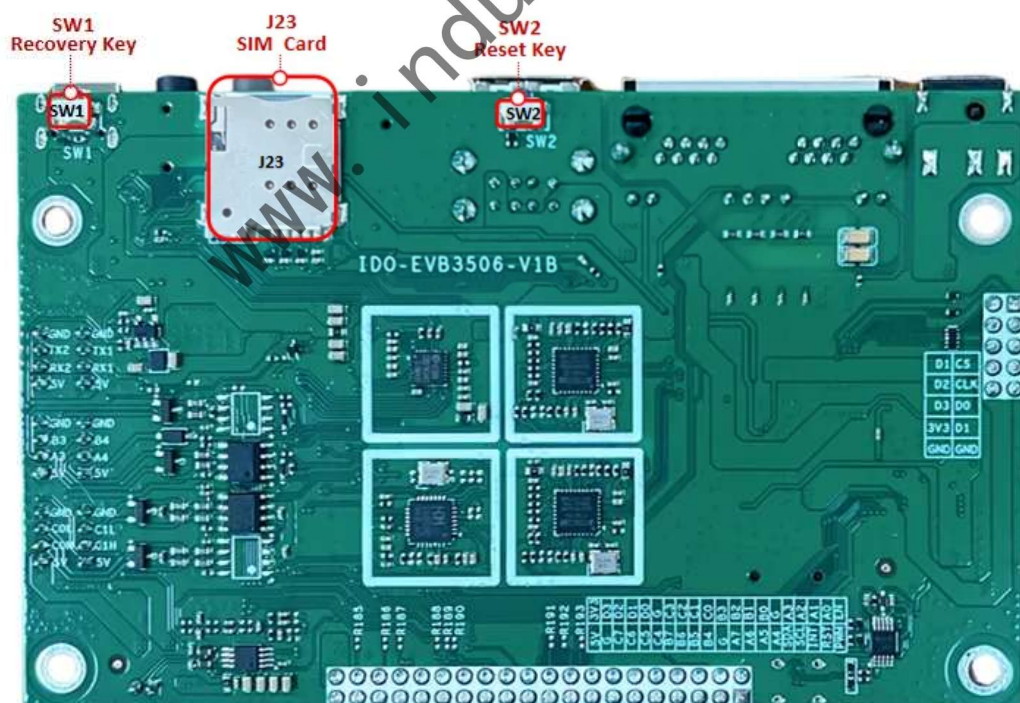
IDO-EVB3506-V1背面接口位号图，如下图所示：
