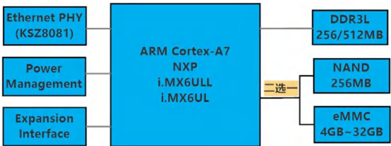
图2. IDO-SOM6Y08 模块逻辑框图
