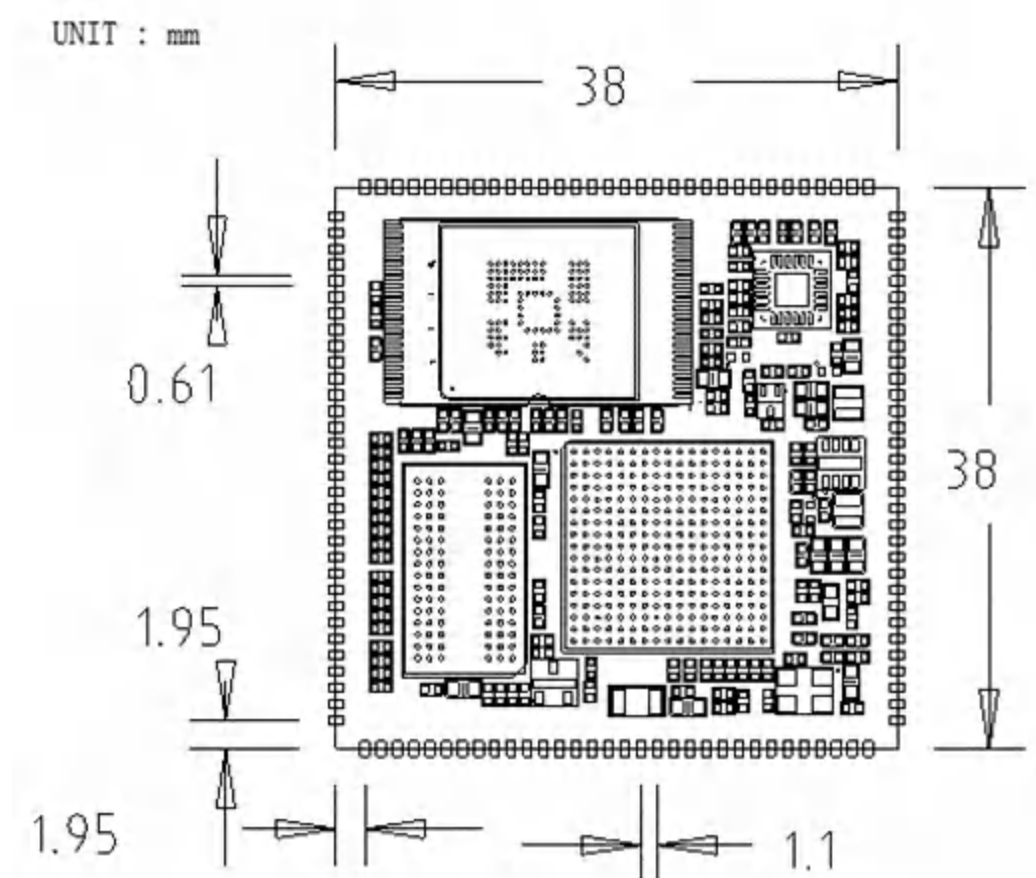
图5. IDO-SOM6Y08 核心板正面尺寸
