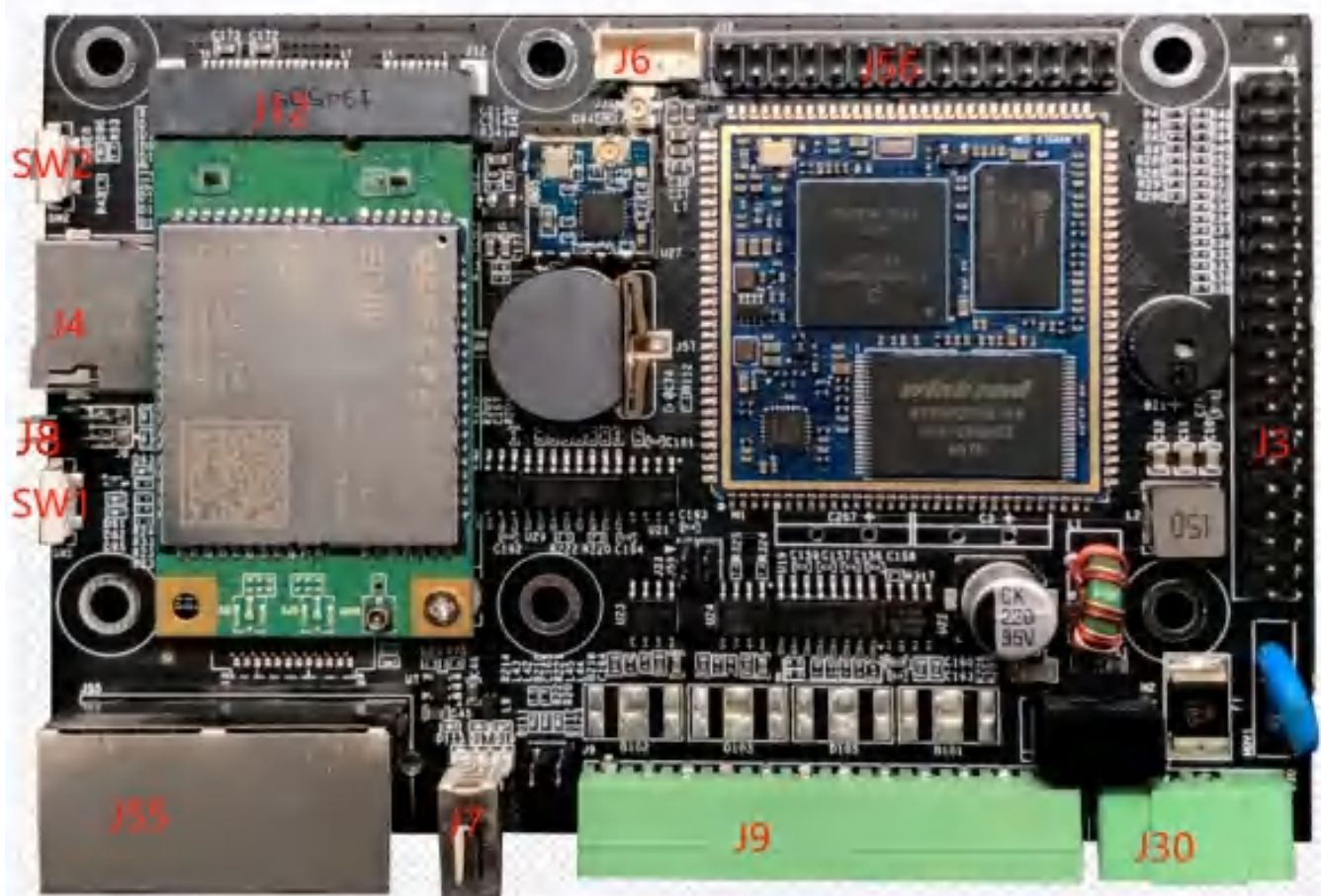
图4. IDO-SBC6Y15正面接口位号图
