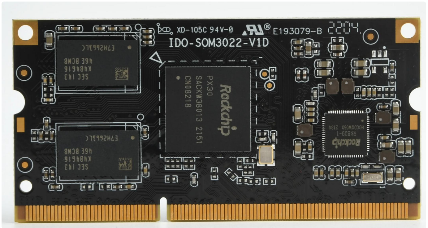
图1. IDO-SOM3022产品示意图
