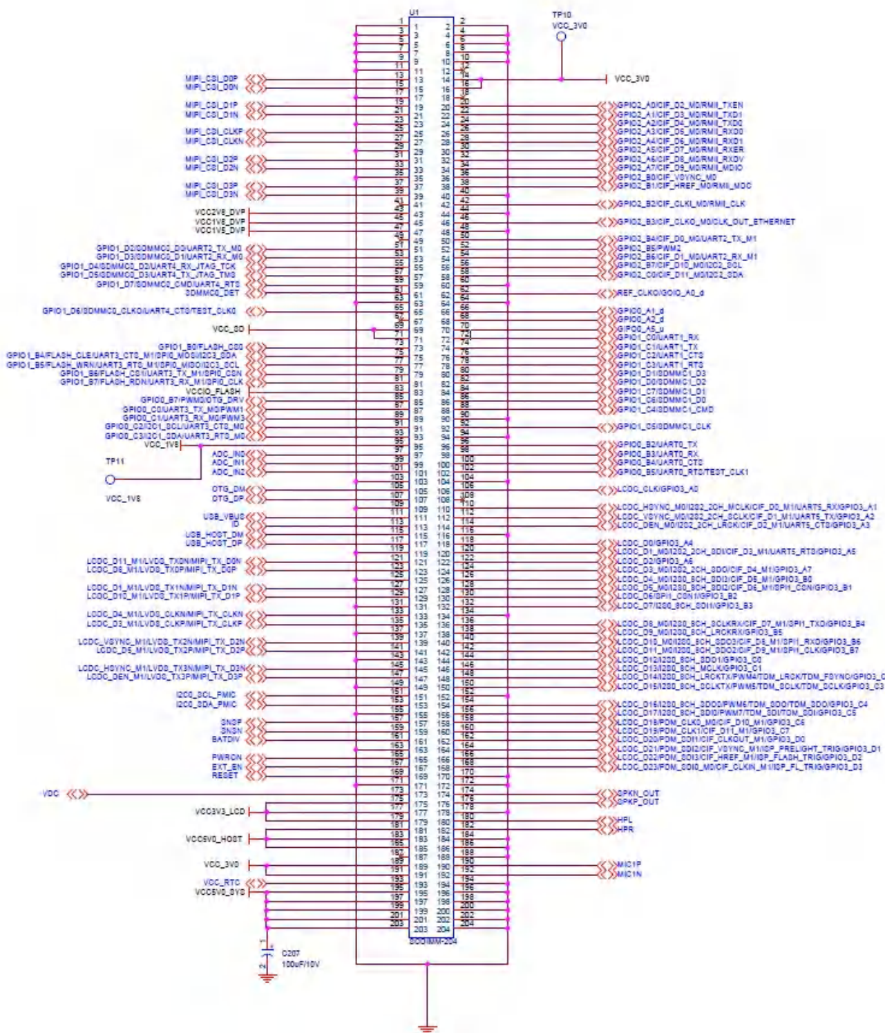
图7. IDO-SOM3022核心板引脚示意图
