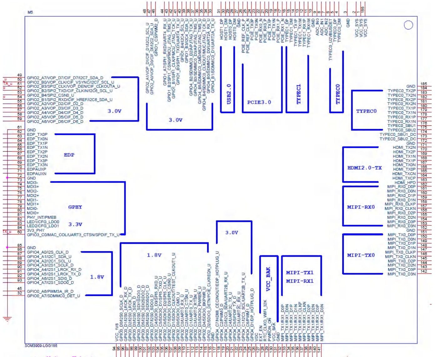
图7. IDO-SOM3909核心板引脚示意图
