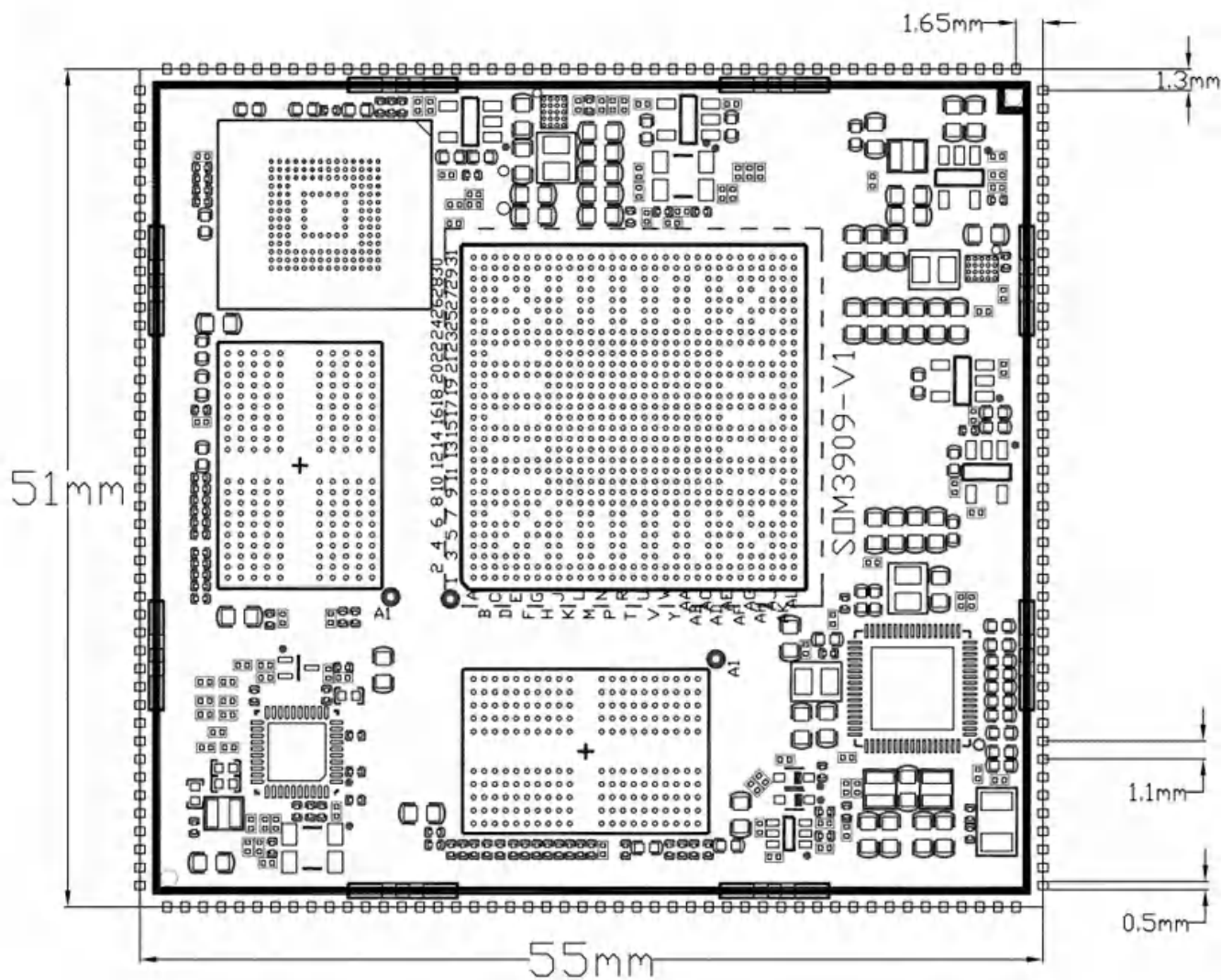
图5. IDO-SOM3909核心板正面尺寸
