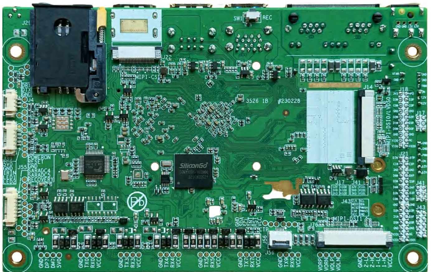
IDO-CTB3526-V1B 正面实物图
