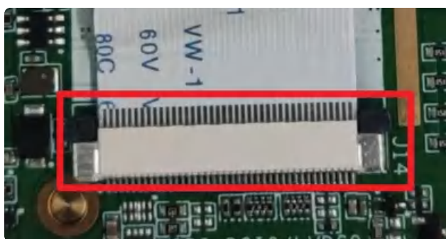
主板LCD排线接线 (排线上接)
