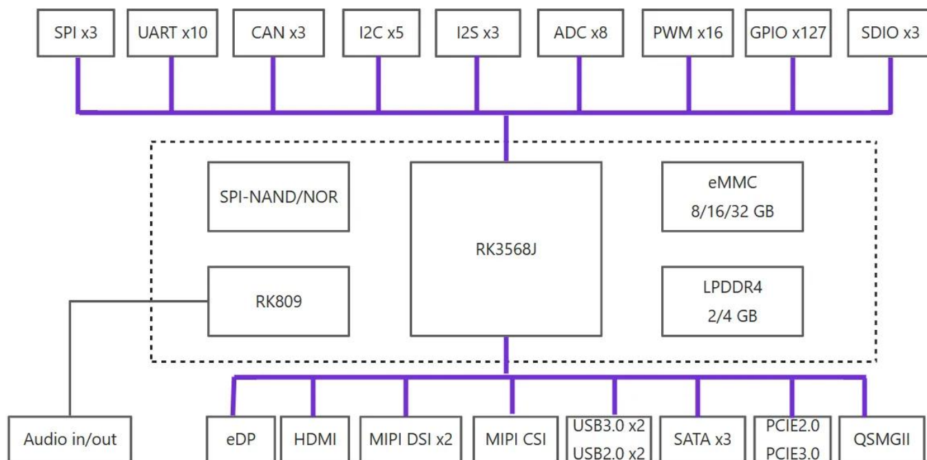
图2. IDO-SOM3568J-V2模块逻辑框图
