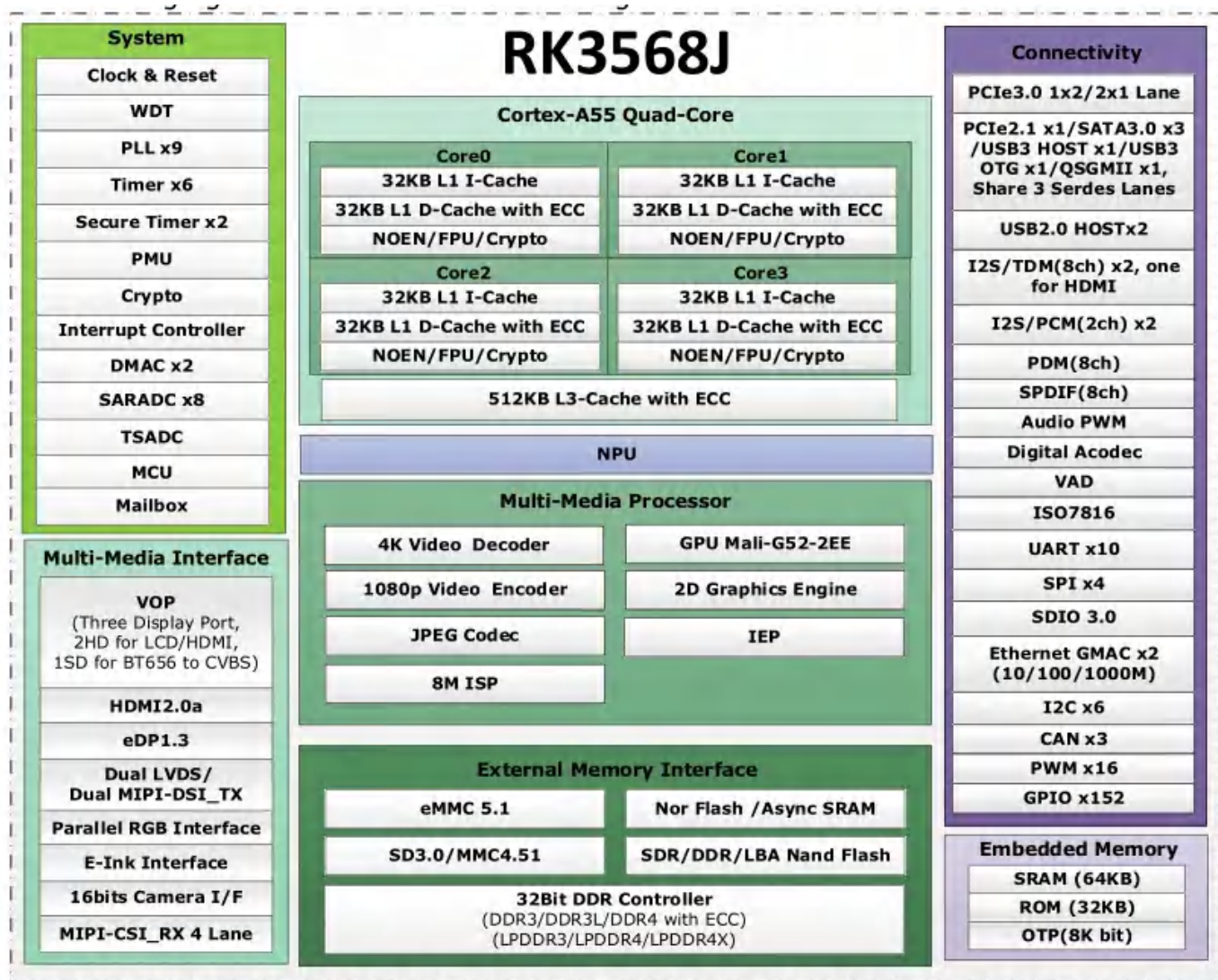
图1. RK3568J SoC框图
