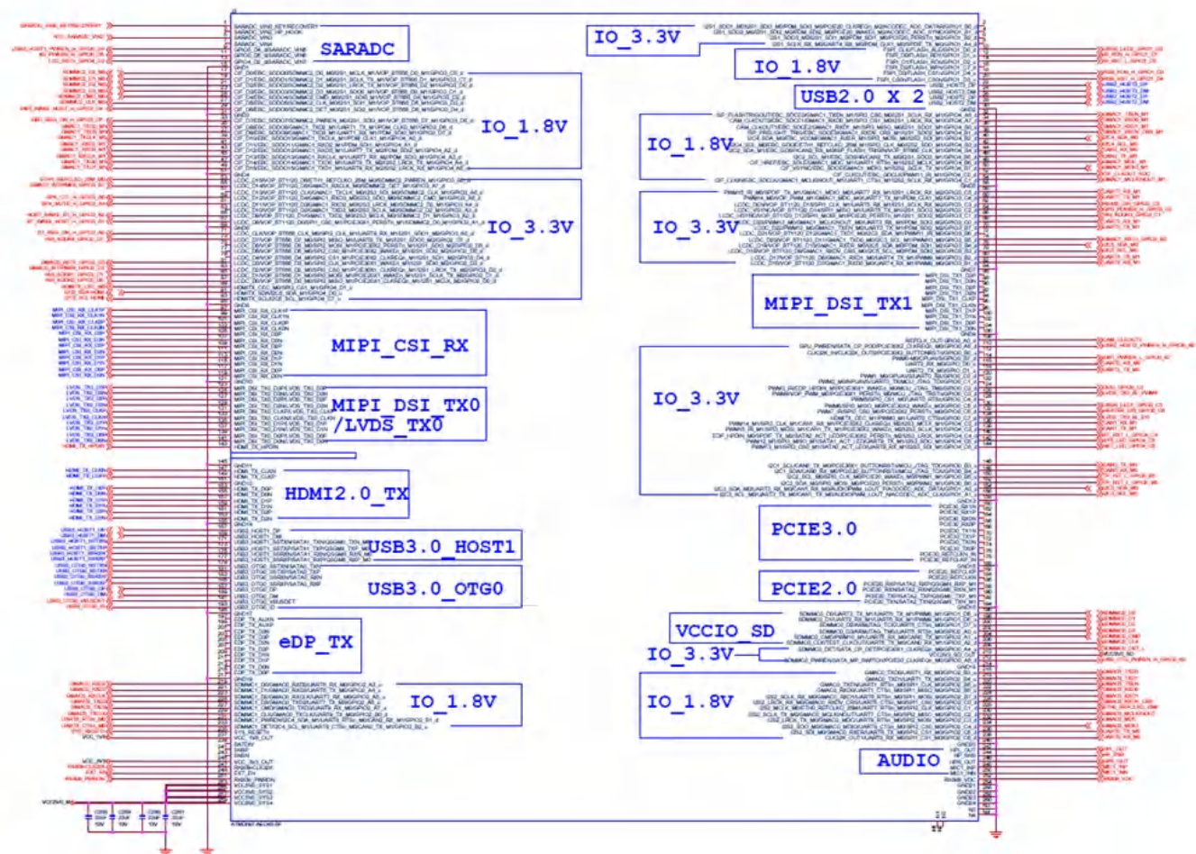
图7. IDO-SOM3568J-V2-E核心板引脚示意图
