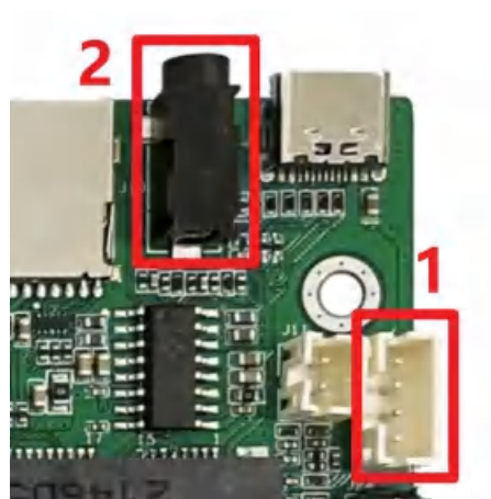
1—喇叭 2—耳机
