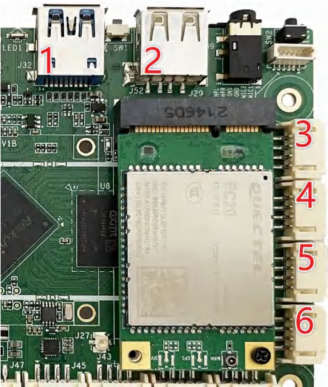
USB接口如上图所示，功能说明如下
