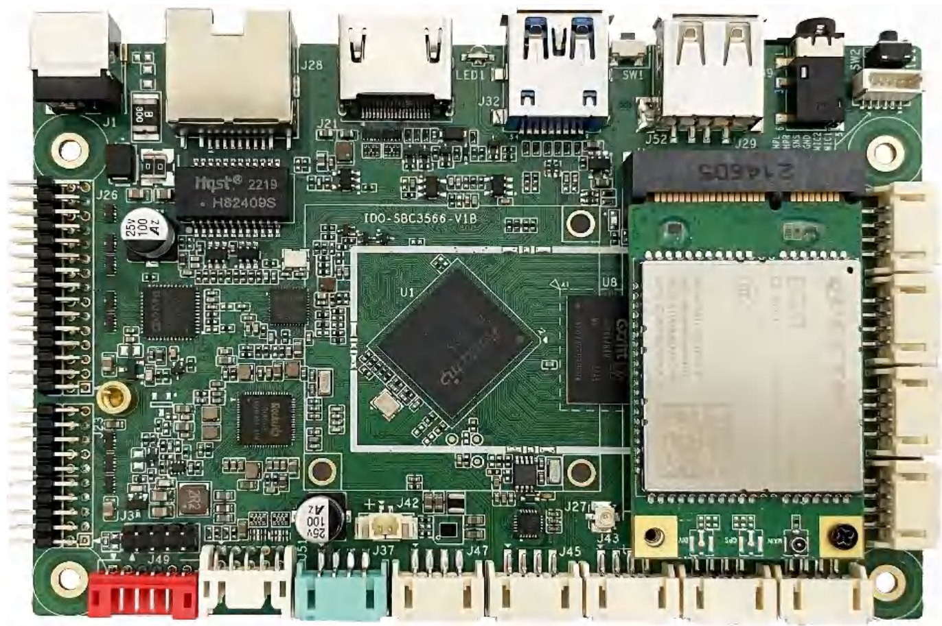
IDO-SBC3566-V1B正面实物图
