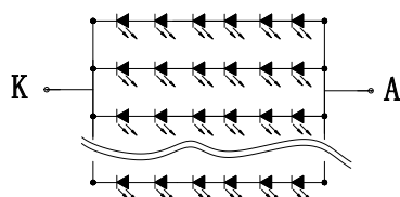
LED电路图 6*6=36LED
