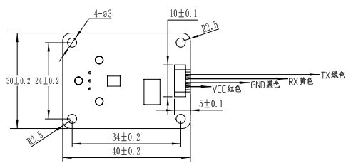
背视图
