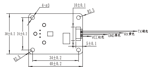
背视图
