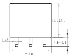
• 正视图
