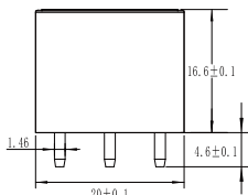
• 正视图
