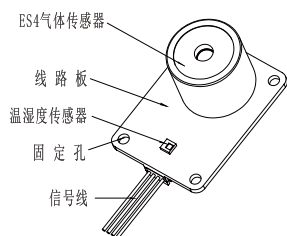
产品示意图
