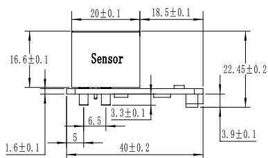
侧视图
