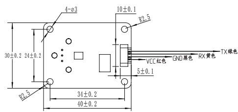
背视图
