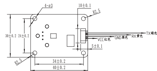
背视图
