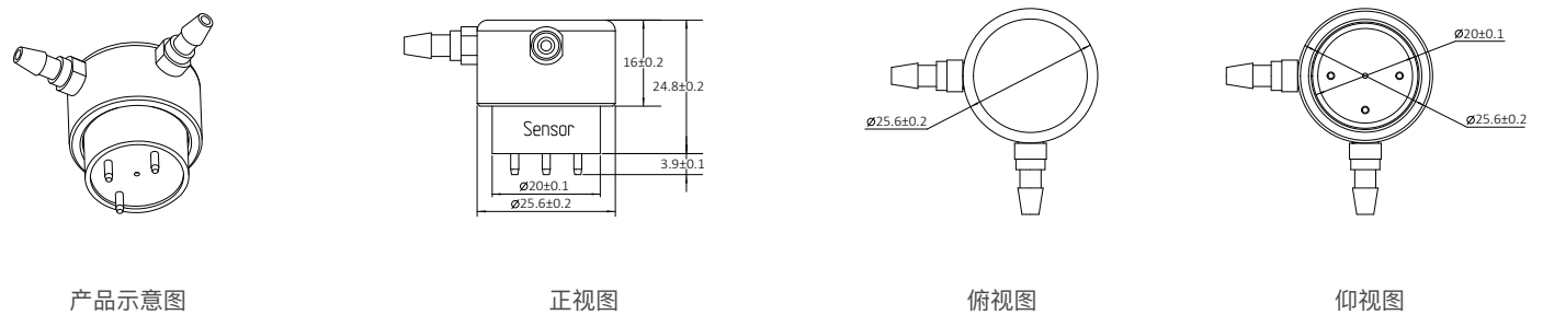
适配ES4/EC4系列传感器结构尺寸示意图 单位：mm
