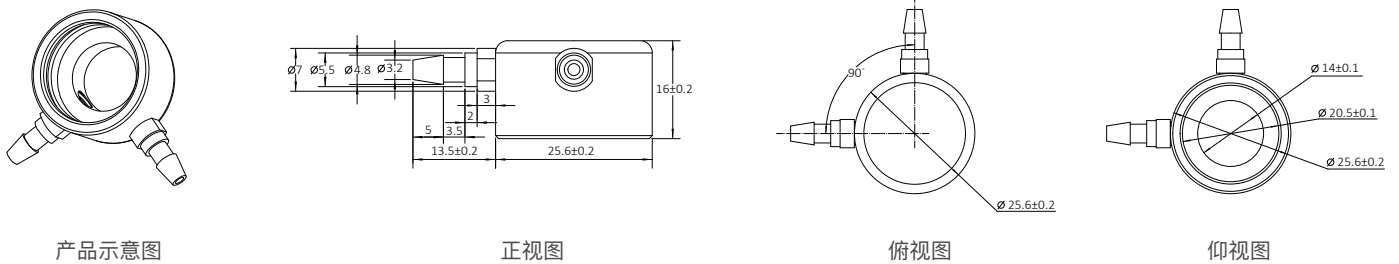
4S 气体传感器流量罩结构尺寸示意图 单位：mm
