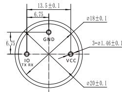
• 仰视图
