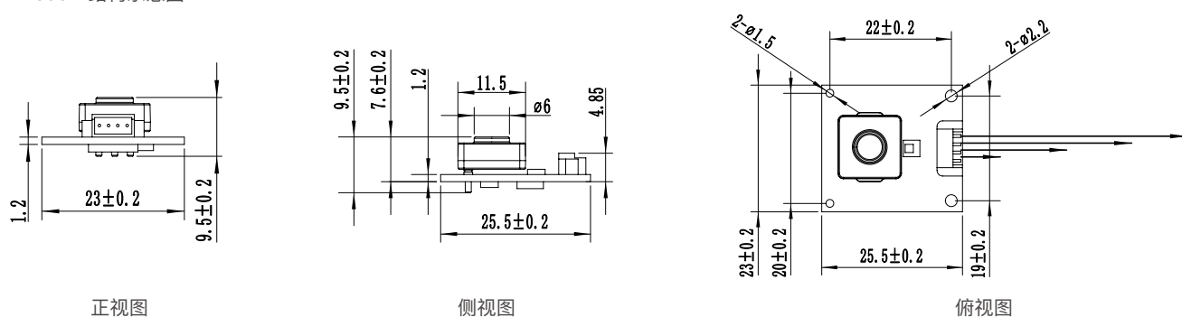
TB600B 结构示意图
