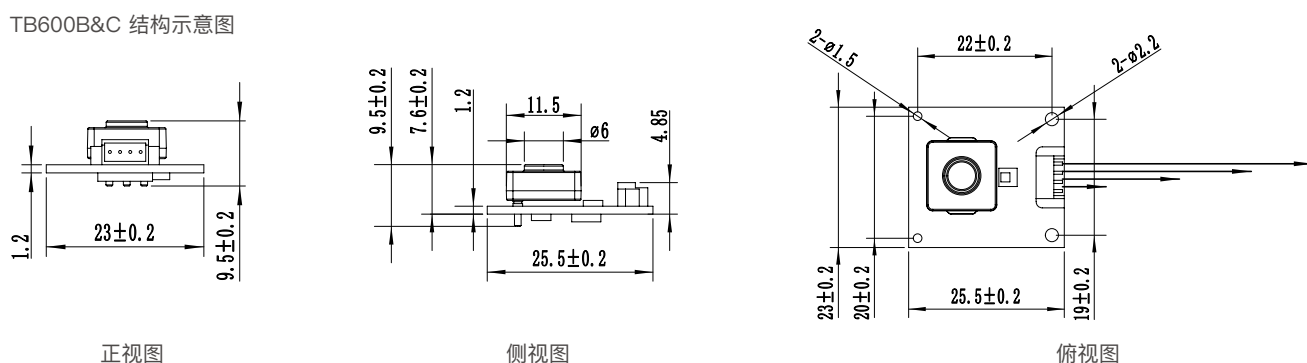
4pin 线结构示意图
