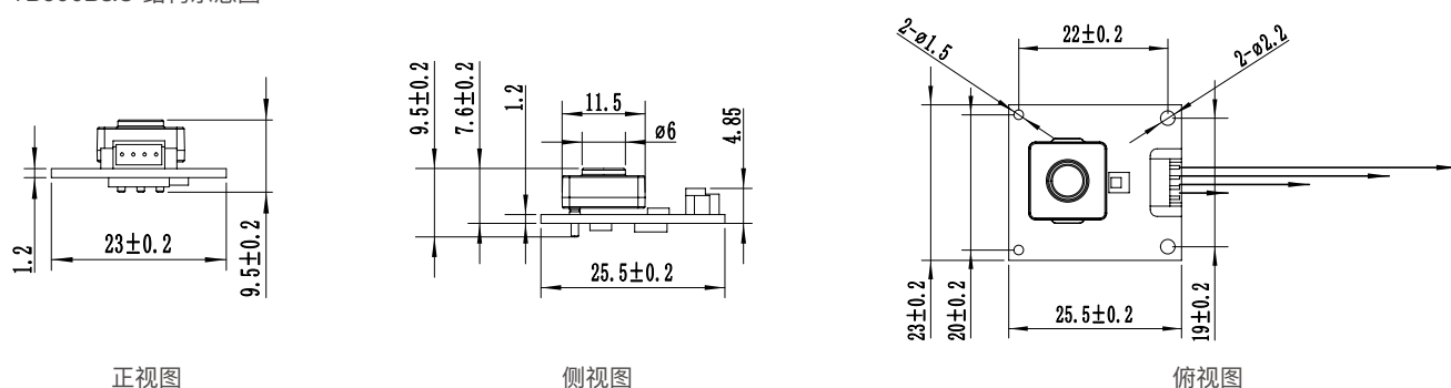
TB600B&C 结构示意图
