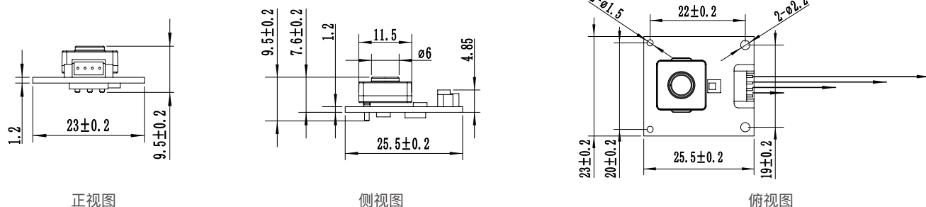
TB600B&C 结构示意图
