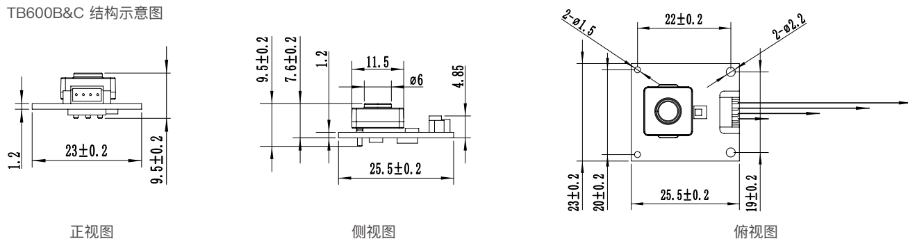
4pin 线结构示意图
