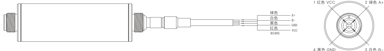
高温版接线图
