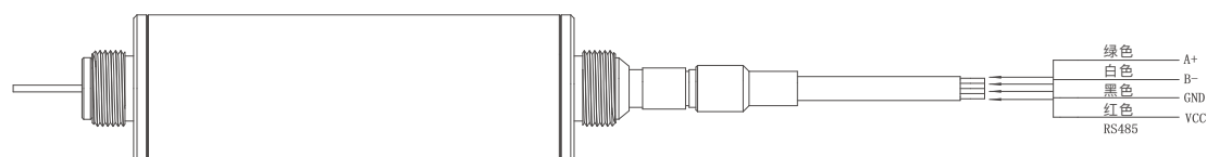
高温版接线图
