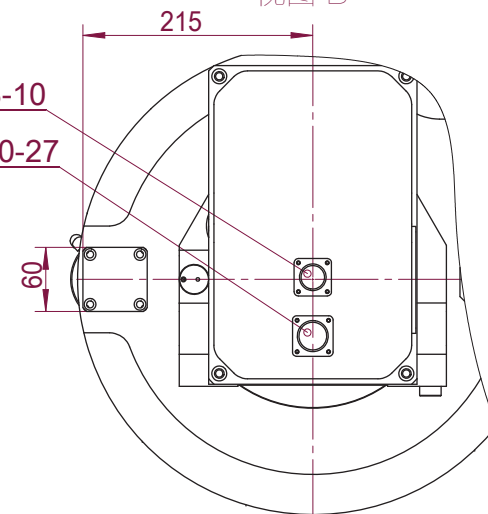
视图 B
