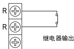
常闭继电器
