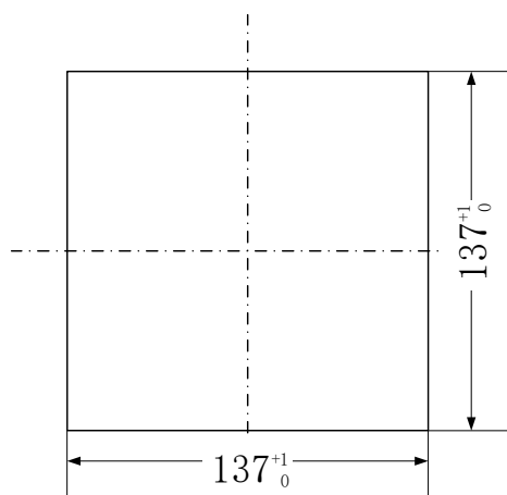
集装表开孔尺寸
