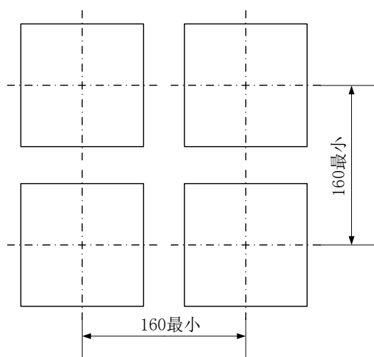
集装表开孔尺寸
