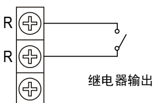
常开继电器
