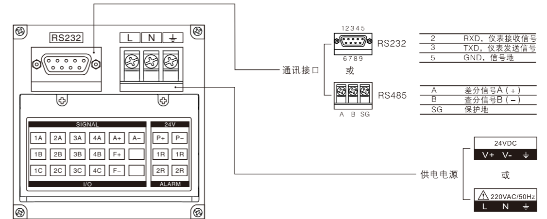
KT100R端子排列
