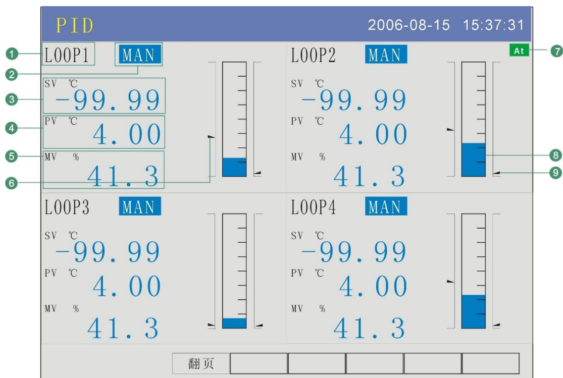
4 路 PID 画面
