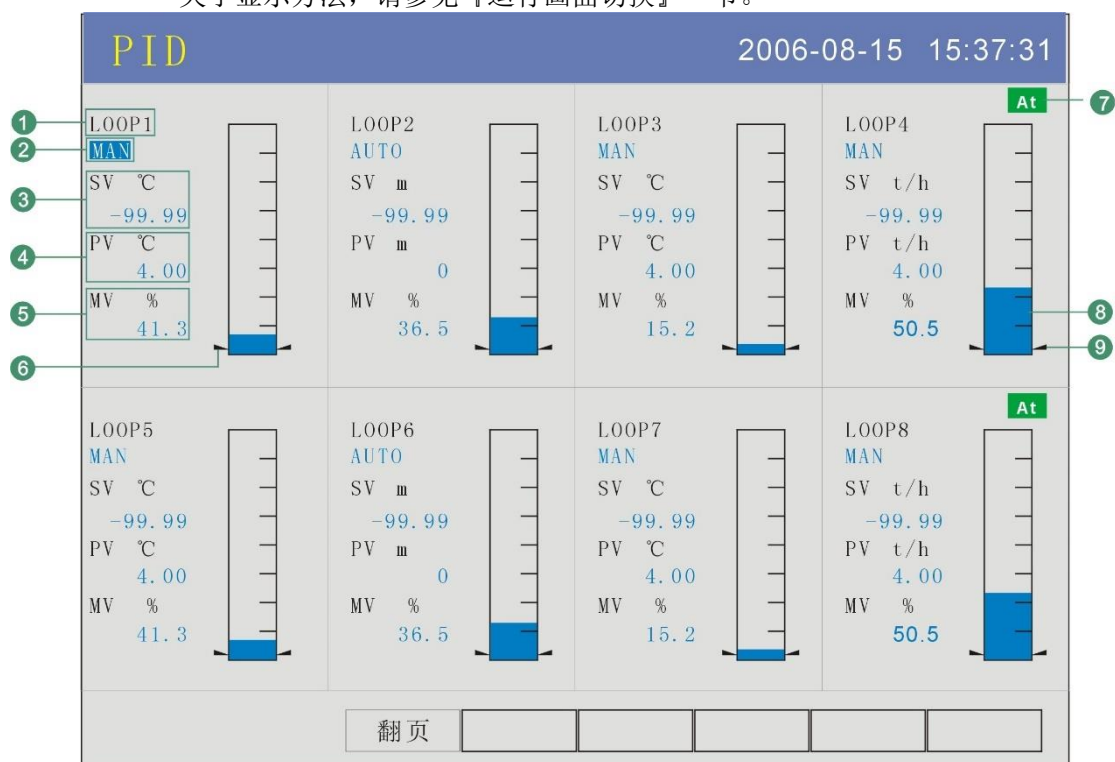
8 路 PID 画面
